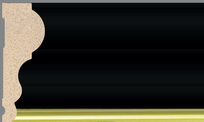
AD-001-S1-A 52 mm x 19 mm
